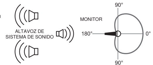
UBICACIONES RECOMENDADAS PARA ALTAVOCES CON MICROFONOS DE CARDIOIDE
