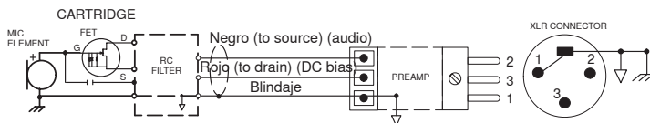
Diagrama de alambrado
